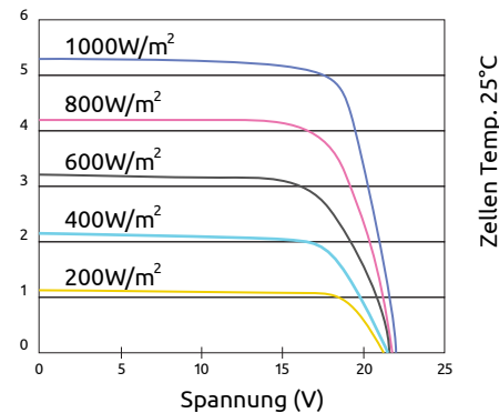
I/U Kurve bei verschiedenen Einstrahlungsstärken
